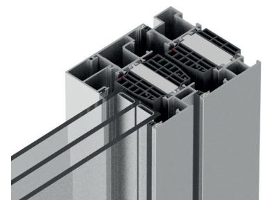
Buiten kader P-19-A100 met inbouwdiepte 91 mm
