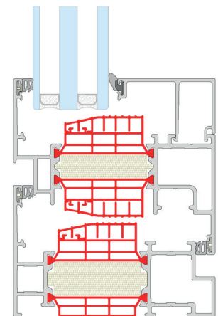
Buiten kader P-19-A100 met inbouwdiepte 91 mm
