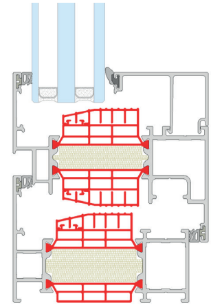
Buiten kader P-19-A120 met inbouwdiepte 82 mm
