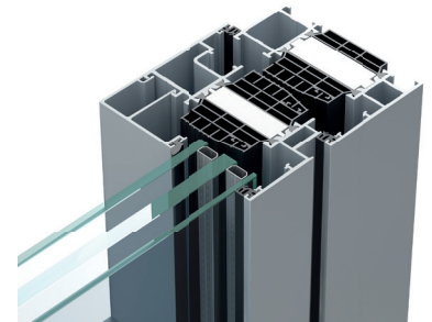
Buiten kader P-19-A120 met inbouwdiepte 82 mm
